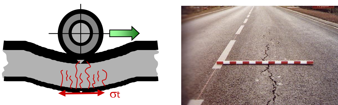
Figure 9 : Mécanisme de fatigue des matériaux traités aux liants hydrauliques et bétons de ciment
