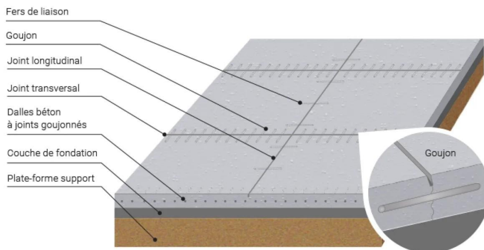
Figure 4 : Disposition des goudjons dans les chaussées en béton
