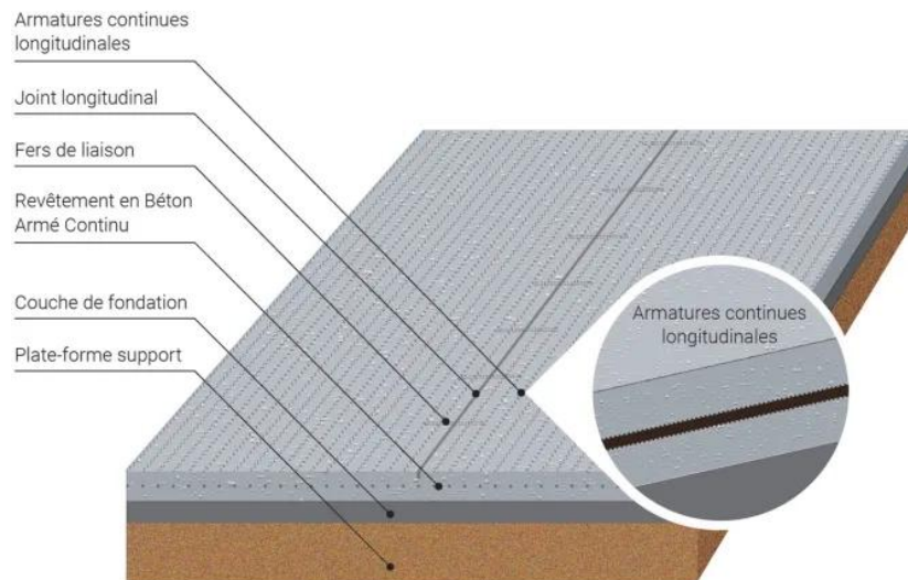
Figure 5 : Disposition des aciers longitudinaux et fers de liasion dans les chaussées en béton
